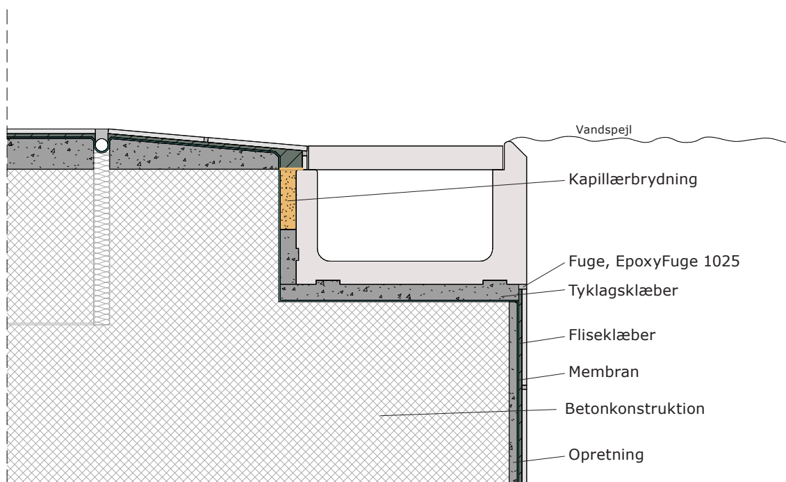
Eksempel på montering af overløbsrende
