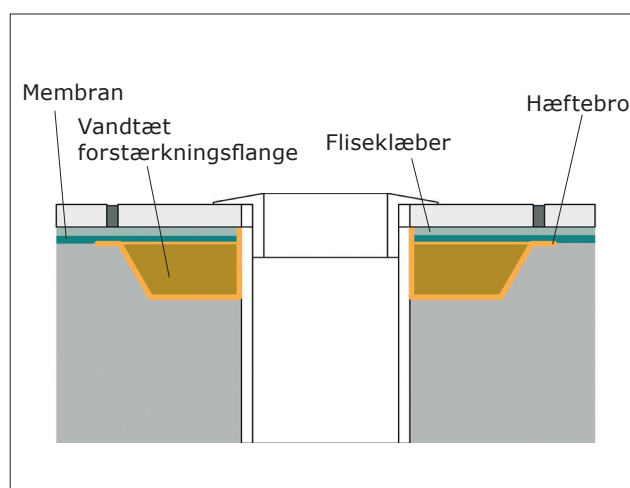
Eksempel på afslutning ved afløb
