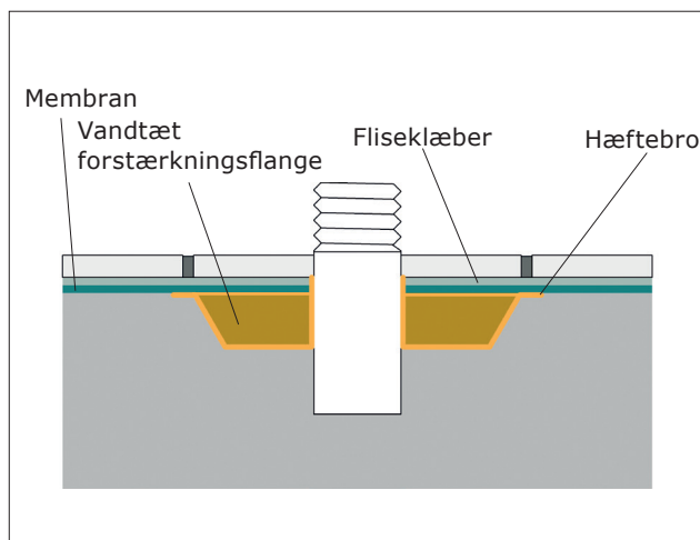
Eksempel på afslutning ved fastgørelsesdetalje
